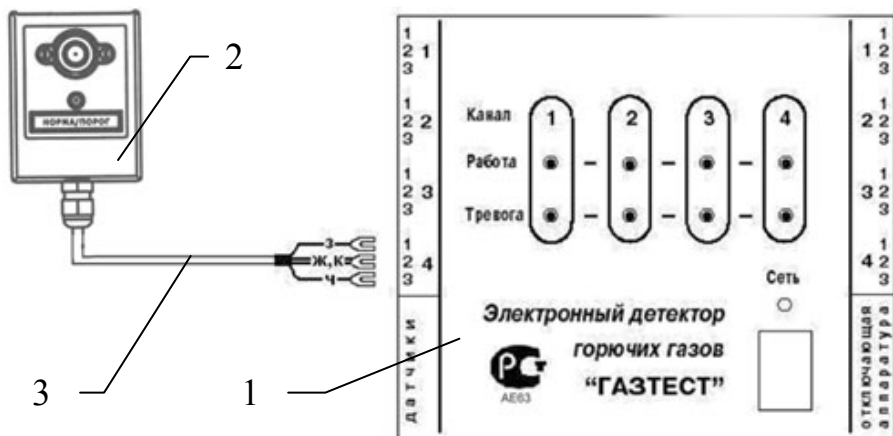
Рис.2. Схема подключения датчика к блоку сигнализации: 1 – передняя панель блока сигнализации; 2 – датчик 4-го канала; 3 – линия связи (буквами обозначен цвет провода): з – зеленый, ж – желтый, к – красный, ч – черный
