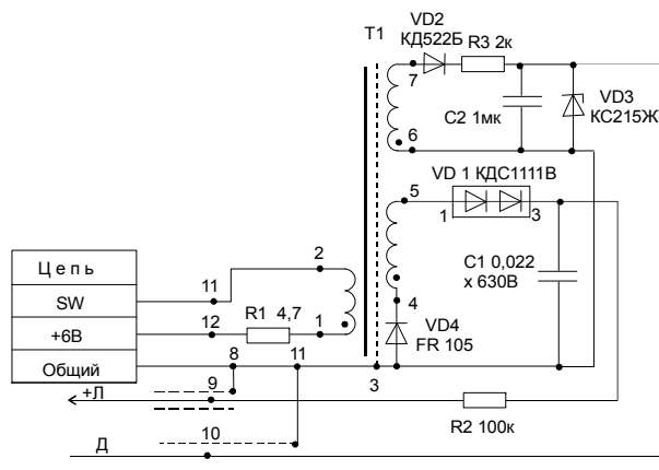
Рис. 4 Электрическая схема искробезопасного высоковольтного блока
