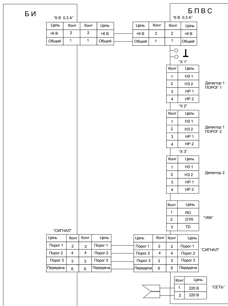
Схема соединения блока измерительного, блока питания и выходных сигналов, внешних устройств.
