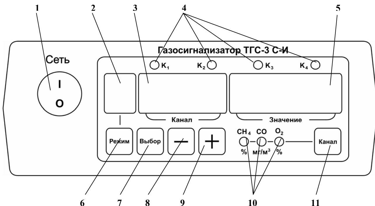
Рисунок 1 Передняя панель блока измерения
